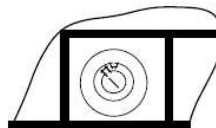
Position du potentiomètre intégré pour un angle initial de 180° / Setting position of the integrated trimmer : 180°
