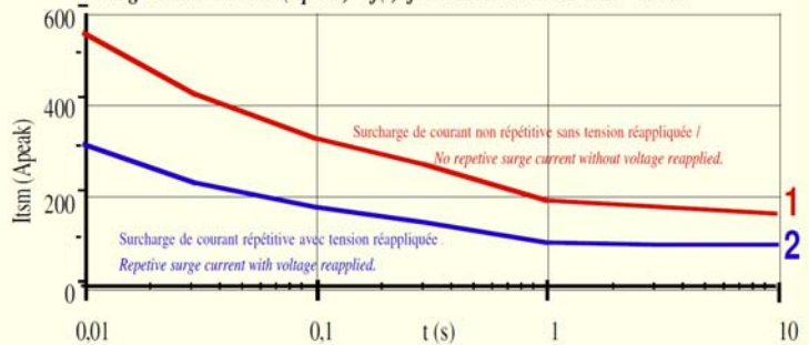
Fig.3 Surcharge de courant : I tsm (Apeak) = f(t) pour modèle 50A(I tsm =550A)
