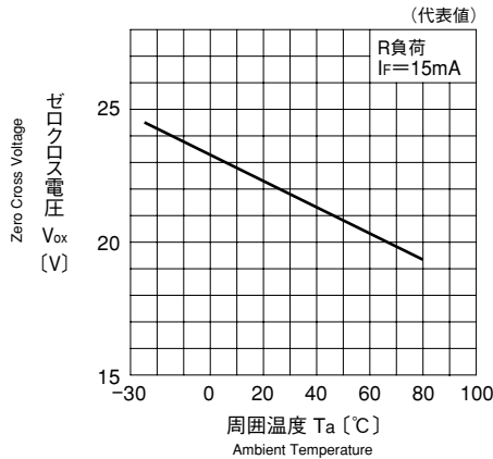
Zero Cross Voltage VS. Ambient Temperature ゼロクロス電圧-周囲温度特性
