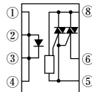
ゼロクロス回路 (JC-MDCタイプに適用)
