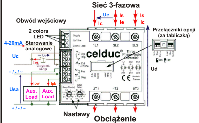
Rys. 4 - Schemat wewnętrzny
