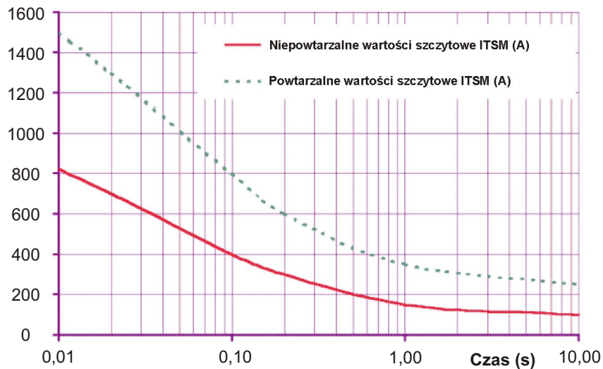
Rys. 8 - Charakterystyka prądu przeciążeniowego
