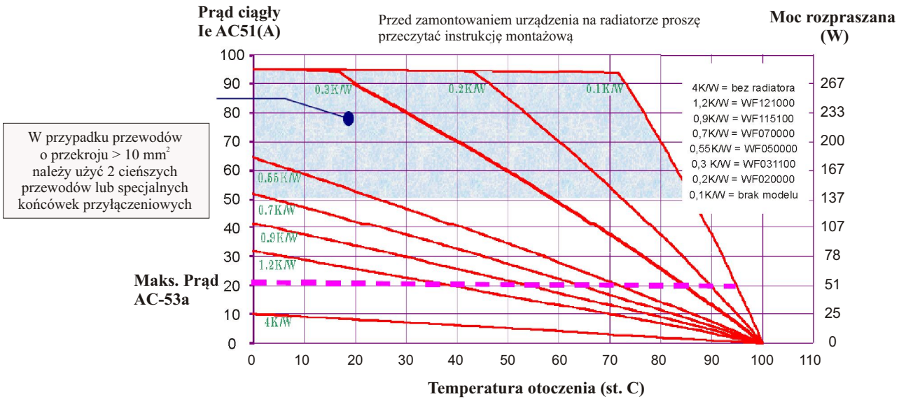
Rys. 8 - Charakterystyka prądu przeciążeniowego
